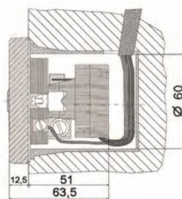
Maßzeichnung: (Einbau-Ansicht)
