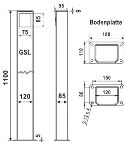
Frontansicht Seitenansicht
