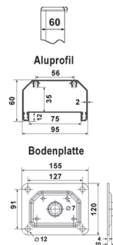
Seitenansicht
