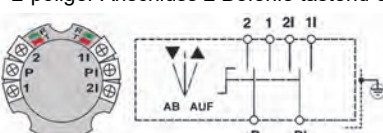
Bild 2 + 5 : S-APZ / EPZ 1-2T(R) 2-poliger Anschluss 2 Befehle tastend o. rastend
