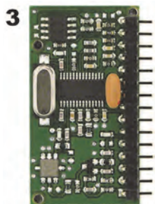
Funkmodul steckbar Maße (LxBxT): 41 x 22 x 10 mm
