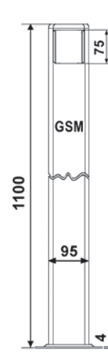
Frontansicht
